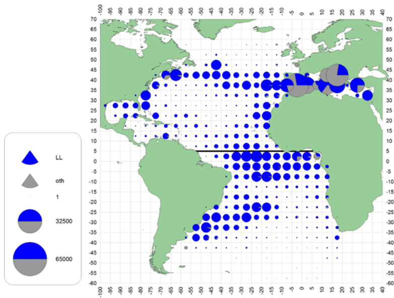
e. SWO (1990-99)
