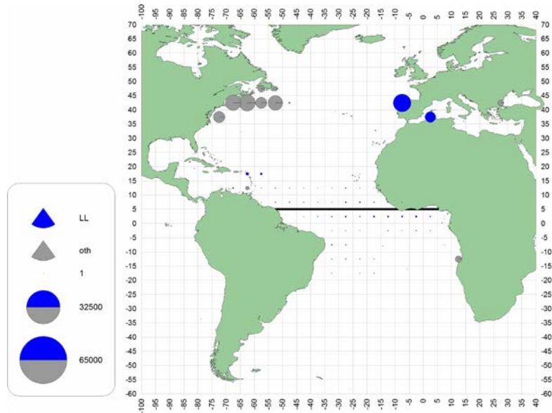
a. SWO(1950-59)
