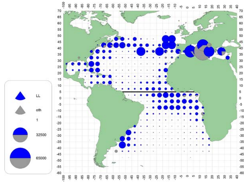
d. SWO (1980-89)
