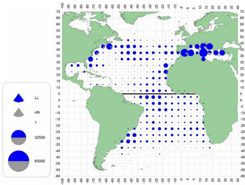
g. SWO (2010-14)
