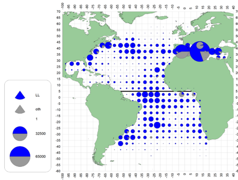
f. SWO (2000-09)
