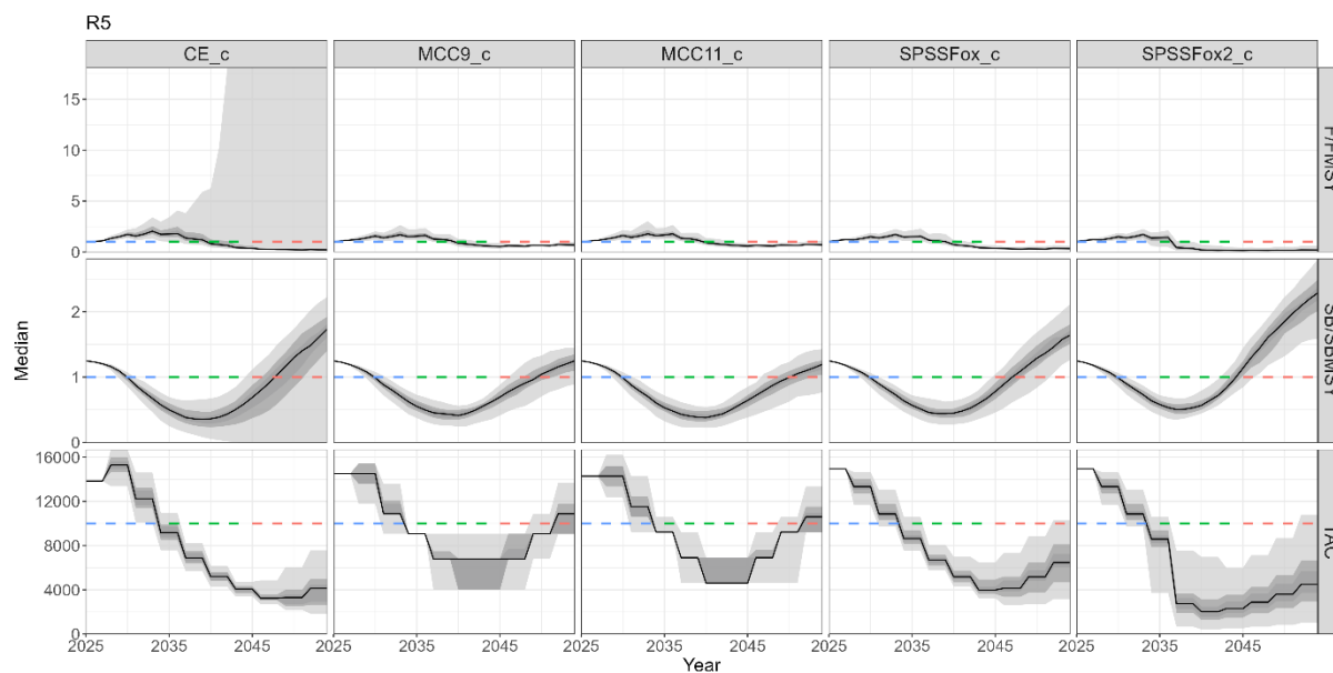
Figura B3. Trayectoria de la mortalidad por pesca (F) con respecto a F_{RMS} (arriba), de la biomasa reproductora (SB) con respecto a SB_{RMS} (centro) y del total admisible de capturas (TAC) para las calibraciones "c" de los CMP según la prueba de solidez frente al cambio climático R5 (presenta un descenso del reclutamiento en los primeros quince años, seguido de una vuelta al reclutamiento medio durante el resto del periodo de proyección). La línea de tendencia negra oscura muestra el valor de la mediana de SB, mientras que los tonos de gris cada vez más claros muestran los percentiles 50, 60 y 90, respectivamente. La línea horizontal de color muestra el objetivo de SB_{RMS} a corto (azul), medio (verde) y largo (rojo) plazo .
