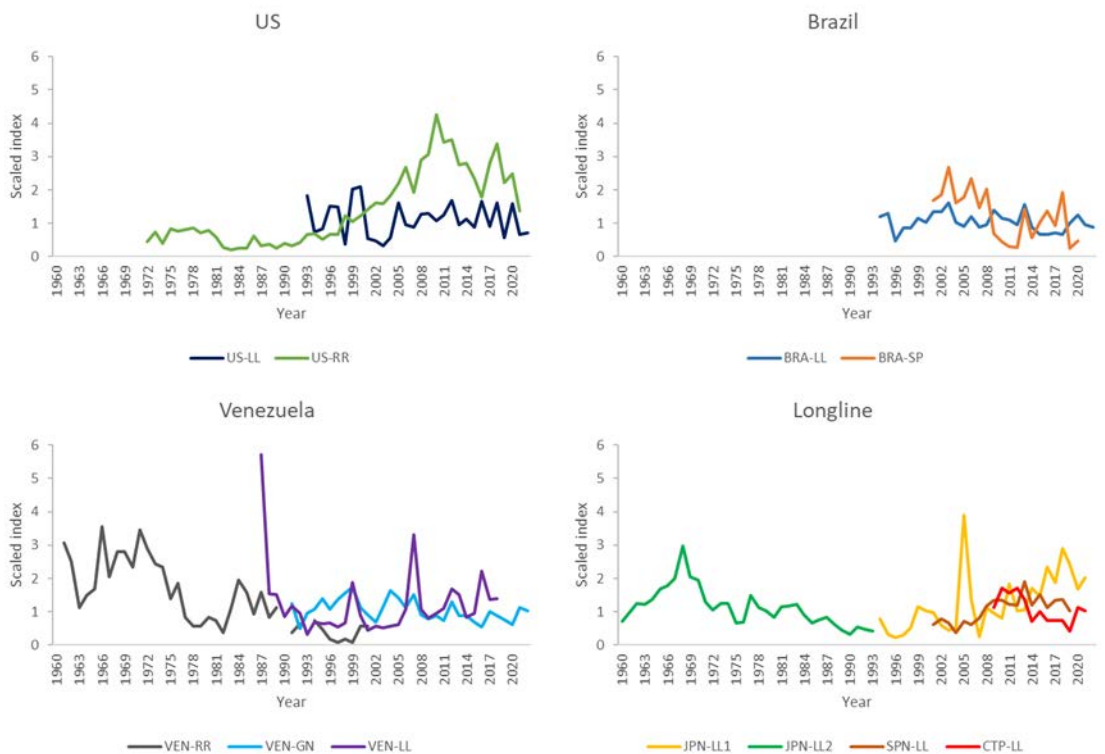
SAI-Figura 4. Índices de abundancia relativa considerados en las evaluaciones de stock de pez vela del Atlántico este y oeste. Todos los índices se han escalado a la media de cada serie antes de hacer el gráfico.
