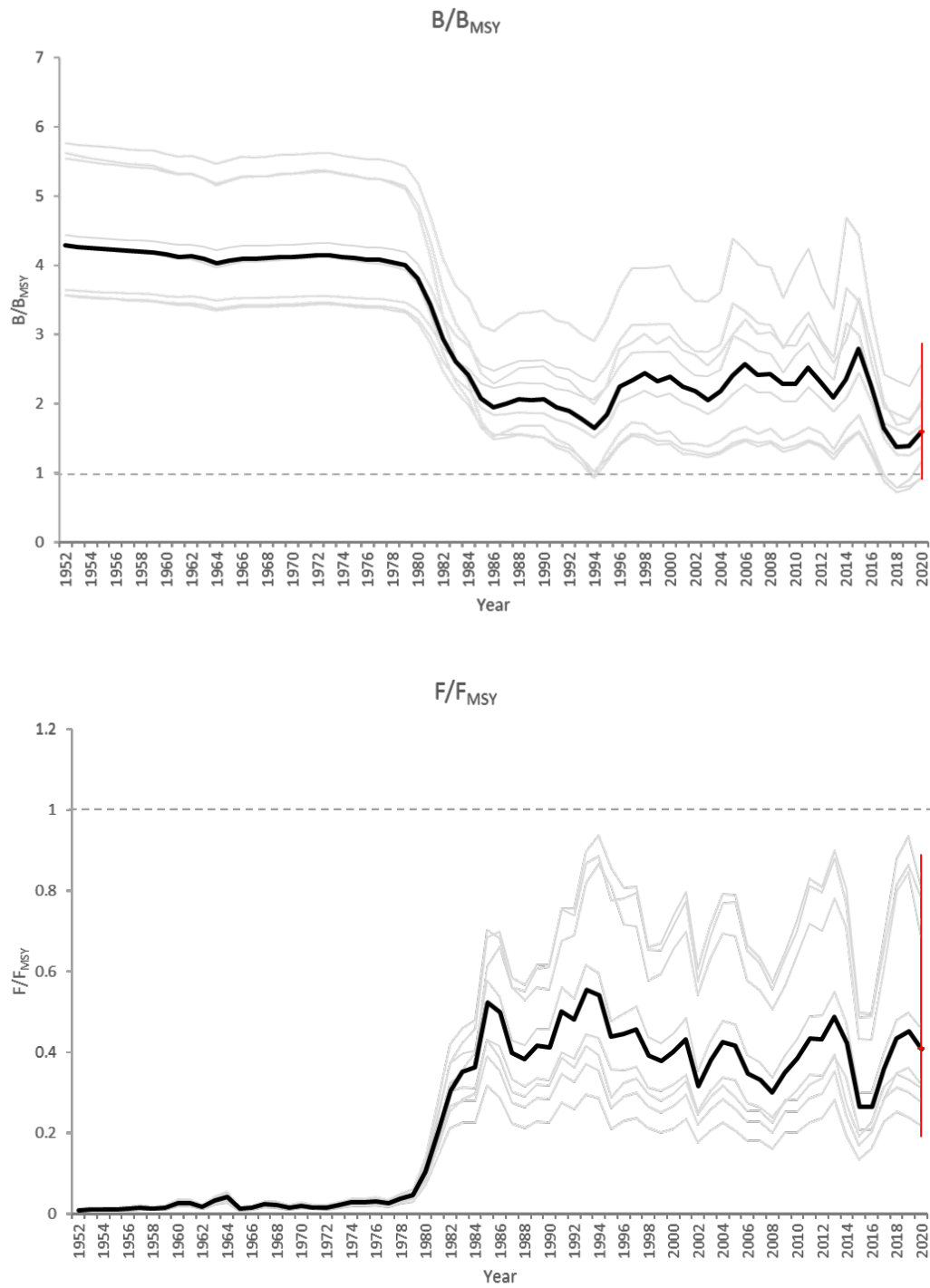
SKJ-Figura 16. SKJ-W Tendencias de la mediana histórica de la abundancia relativa ( B/B_{RMS} ) (superior) y de la mortalidad por pesca ( F/F_{RMS} ) (inferior) para el stock de listado del oeste estimadas por cada modelo de la matriz de incertidumbre; la línea continua representa la mediana de las tendencias trazadas y la línea roja vertical en 2020, el límite de confianza del 95 % de los resultados estocásticos combinados.
