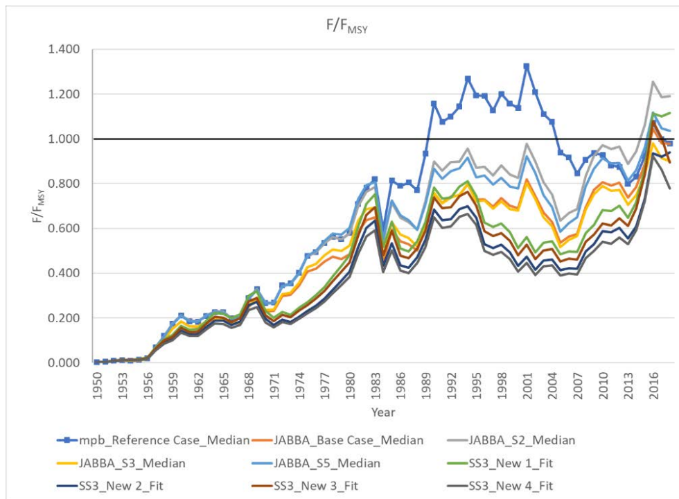
YFT-Figure 10. Estimaciones de la mortalidad por pesca relativa ( F/F_{RMS} ) obtenida para todos los ensayos del modelo utilizados para desarrollar el asesoramiento de ordenación.
