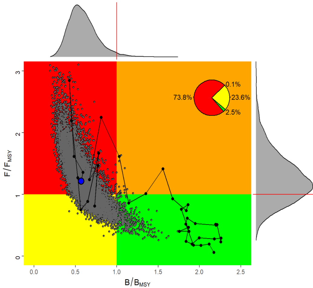
ALB-MD-Figura 4. Atún blanco del Mediterráneo: trayectorias del estado del stock de B/B_{MSY} y F/F_{RMS} a lo largo del tiempo (1980-2019), así como incertidumbre en la estimación actual (diagramas de Kobe) para el modelo de producción excedente bayesiano y probabilidad de estar sobrepescado y experimentando sobrepesca (rojo, 73,8 %), de no estar sobrepescado ni experimentando sobrepesca (verde, 2,5 %), de estar sobrepescado pero no experimentando sobrepesca (amarillo, 23,6 %) y de estar experimentando sobrepesca pero no estar sobrepescado (naranja, 0,1 %). Las distribuciones de probabilidad mostradas en cada eje representan la incertidumbre en torno a las actuales B/B_{RMS} y F/F_{RMS} .
