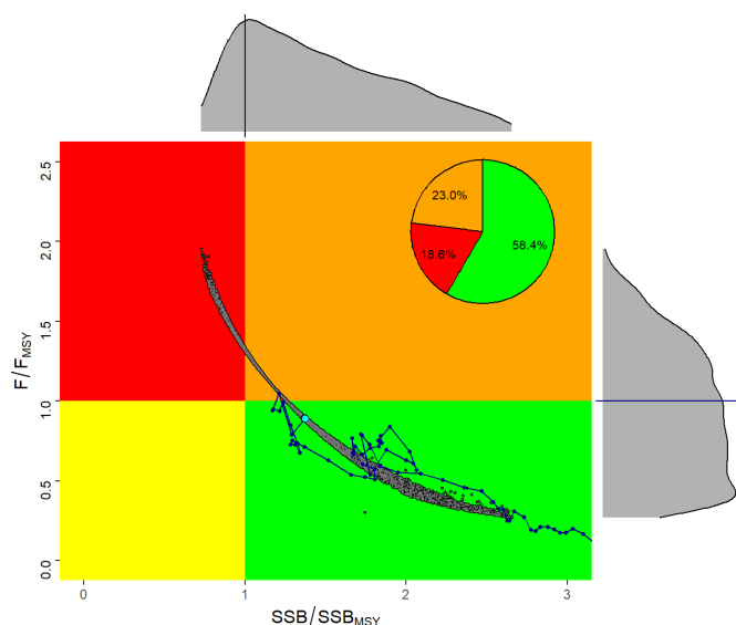
Figure 1. Diagramme de Kobe pour l'état du stock d'albacore de l'Atlantique en 2022, estimé lors de l'évaluation du stock d'albacore de 2024 (Anon., 2024k). Les points gris représentent les 4.000 scénarios du modèle Stock Synthesis ; le cercle bleu est la médiane de ces scénarios et les histogrammes marginaux représentent la distribution de SSB/SSB_{PME} ou F/F_{PME} . La ligne noire indique la trajectoire de l'état du stock à partir de 1958. Le diagramme circulaire inséré indique la probabilité que le stock se situe dans chaque quadrant de couleur de Kobe. Les distributions de probabilité indiquées sur chaque axe représentent l'incertitude entourant B/B_{PME} et F/F_{PME} actuelles.
