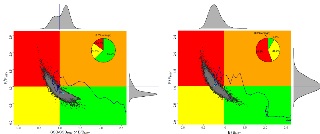
Figure 1. Diagramme de Kobe pour l'état du stock d'espadon de l'Atlantique Nord (à gauche) et Sud (à droite) en 2020, estimé lors de l'évaluation des stocks de 2022. Les diagrammes circulaires insérés indiquent la probabilité que le stock se situe dans chaque quadrant de couleur de Kobe. Les distributions de probabilités indiquées dans chaque axe représentent l'incertitude autour des B/B_{PME} et F/F_{PME} actuelles. La ligne noire indique la trajectoire de l'état du stock à partir de 1950.
