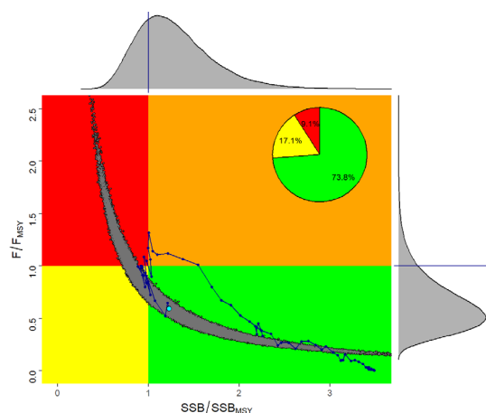
Figure 1. Diagramme de Kobe pour l'état du stock de thon obèse de l'Atlantique en 2023, estimé lors de l'évaluation du stock de 2025. La ligne indique la trajectoire de l'état du stock à partir de 1950. Le diagramme circulaire inséré indique la probabilité que le stock se situe dans chaque quadrant de couleur de Kobe.
