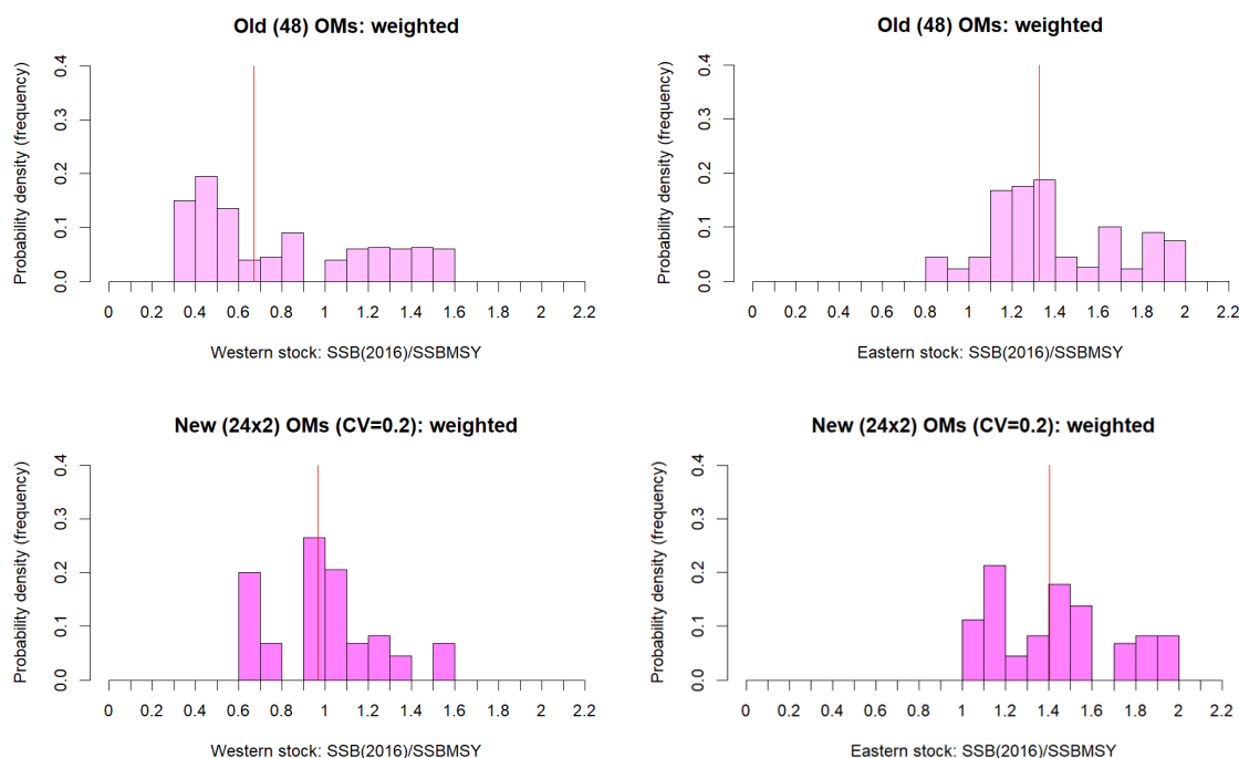
Figure 19.11.3. Diagrammes de l'état du stock de 2016 pour le stock de l'Ouest (en haut à gauche : les 48 OM originaux utilisés dans la MSE de 2022 ; en bas à gauche : les 24 OM reconditionnés intégrant les résultats de CKMR de l'Ouest) et le stock de l'Est (en haut à droite : les 48 OM originaux utilisés dans la MSE de 2022 ; en bas à droite : les 24 OM reconditionnés intégrant les résultats de CKMR de l'Ouest). La ligne verticale rouge est la médiane des OM.
