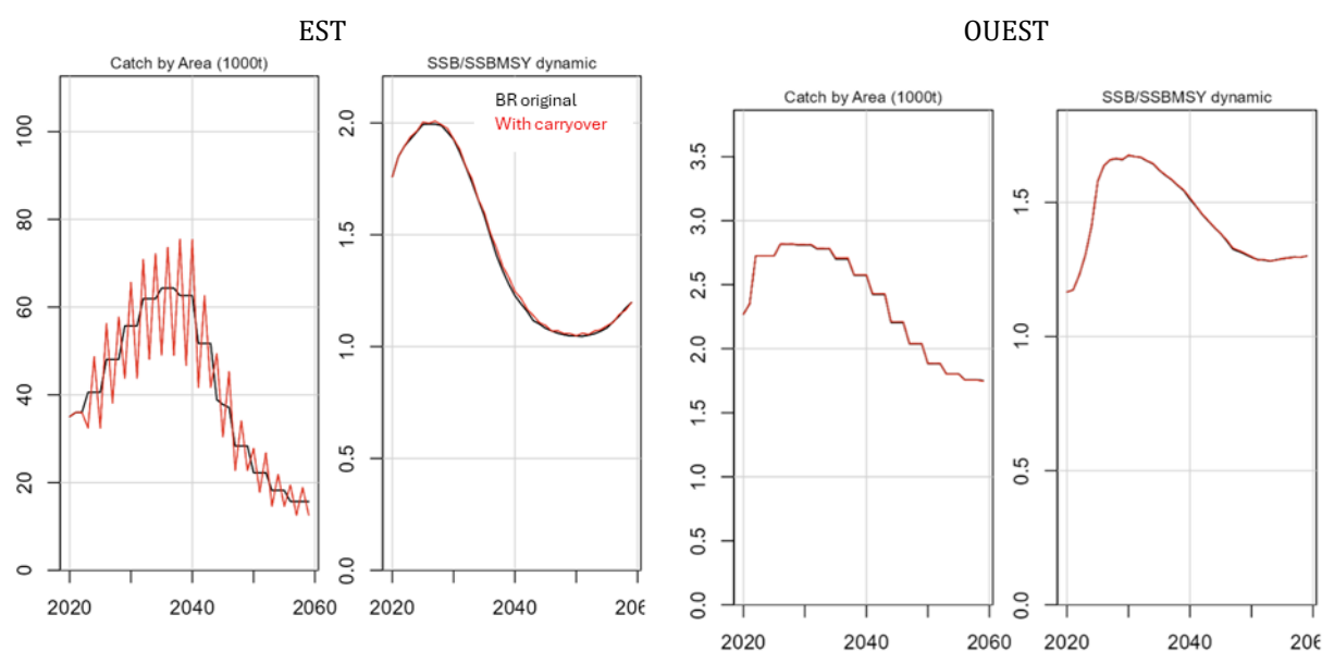
Figure 19.14.1 Projections des captures médianes (par zone) et de la SSB (par stock) mises à la moyenne sur tous les OM de la grille et simulations répliquées pour la MP adoptée : cas de base original en noir et avec le report en rouge.
