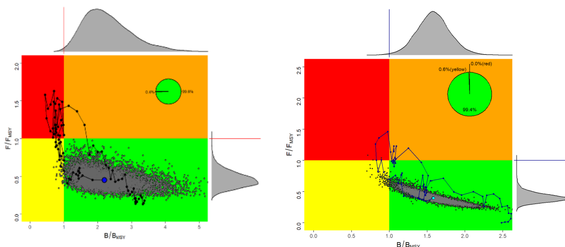
Figure 1. Diagramme de Kobe pour l'état des stocks de germon de l'Atlantique Nord (à gauche) et Sud (à droite) en 2021 et 2018, respectivement. Le diagramme de l'Atlantique Nord montre la trajectoire de l'état du stock de 1930 à 2021, et celui de l'Atlantique Sud de 1958 à 2018, telle qu'elle a été estimée lors de l'évaluation du stock de 2023 (Anon., 2023a) et l'évaluation du stock de 2020 (Anon., 2020a), respectivement. La ligne, dans les deux diagrammes, indique la trajectoire de l'état du stock à partir de 1930 et 1958, respectivement. Le diagramme circulaire inséré indique la probabilité que le stock se situe dans chaque quadrant de couleur de Kobe.
