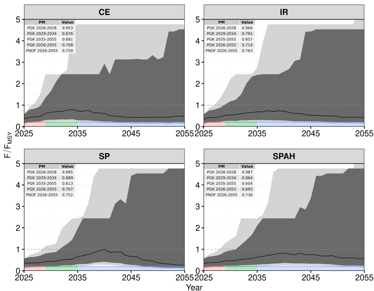
Figure 19.42.3. Projection de la mortalité par pêche par rapport à la F_{PME} ( F/F_{PME} ) pour le listao de l'Atlantique Ouest dans le cadre de quatre CMP, projetées pour la période 2026-2055. La ligne noire représente la trajectoire médiane, tandis que les zones ombrées correspondent aux quantiles de 80% et 95% respectivement. La ligne horizontale en pointillé rouge indique F_{PME} = 1 . Les barres colorées en bas indiquent la référence de la période de projection temporelle (couleur rouge : courte ; couleur verte : moyenne ; couleur bleue : longue).
