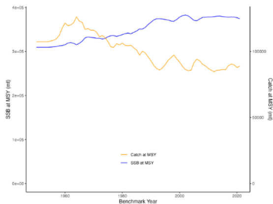
Figure 2. SSB PME dynamique et prises au niveau de la PME indiquant les effets des changements de sélectivité pour le thon obèse.
