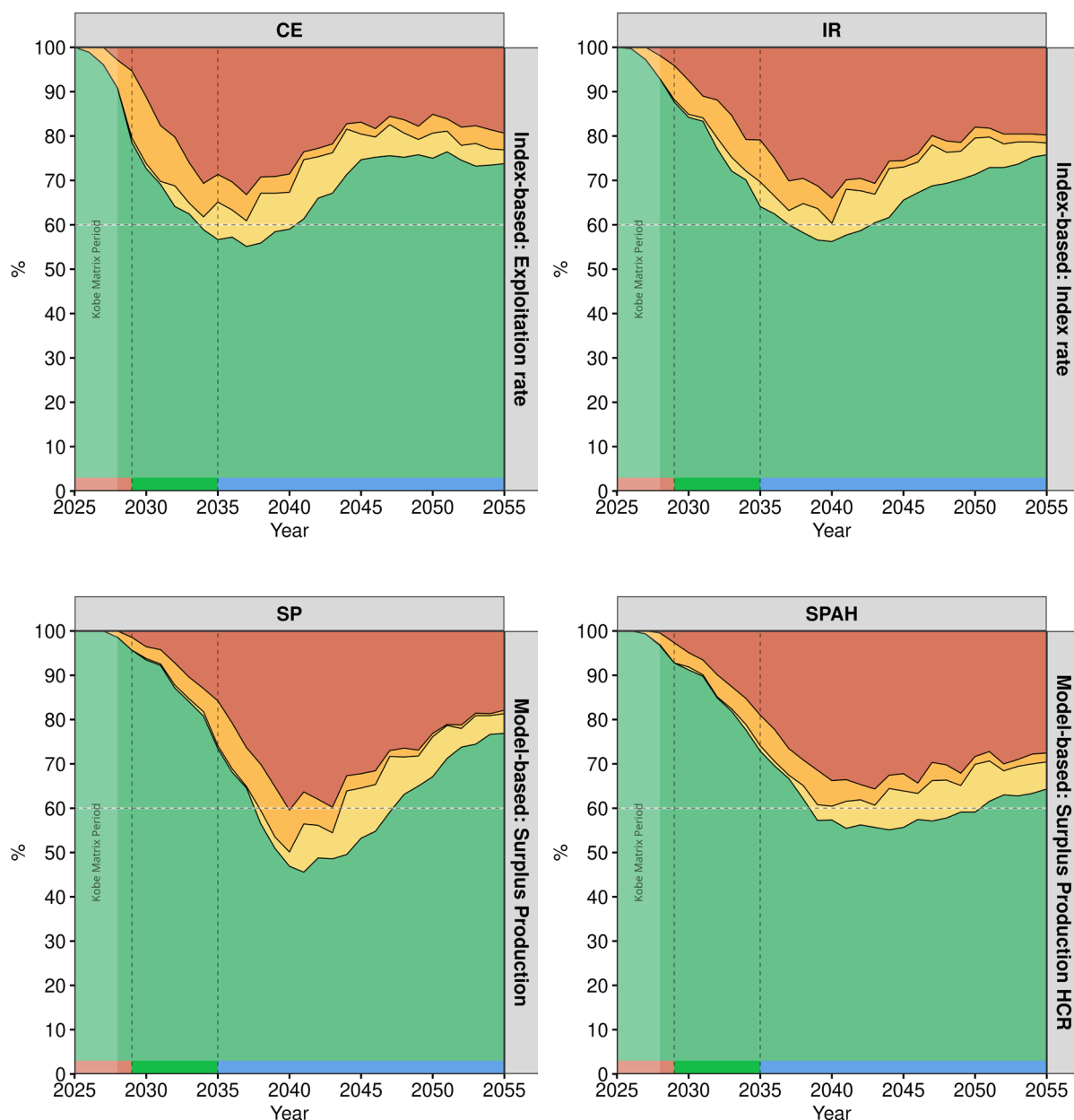
Figure 19.42.5. Diagramme temporel de Kobe montrant le pourcentage (axe vertical) des simulations de tous les OM de référence qui se situent dans chacun des quadrants de Kobe pour chaque année de projection (axe horizontal). Le vert indique que le stock n'est ni surexploité ni ne fait l'objet de surpêche. L'orange signifie que le stock fait l'objet de surpêche mais n'est pas surexploité. Le jaune indique que le stock est surexploité mais ne fait pas l'objet de surpêche. Le rouge signifie que le stock est à la fois surexploité et fait l'objet d'une surpêche continue. La ligne verticale délimite les différentes périodes temporelles, les barres rouges représentant le court terme, les vertes le moyen terme et les bleues le long terme.
