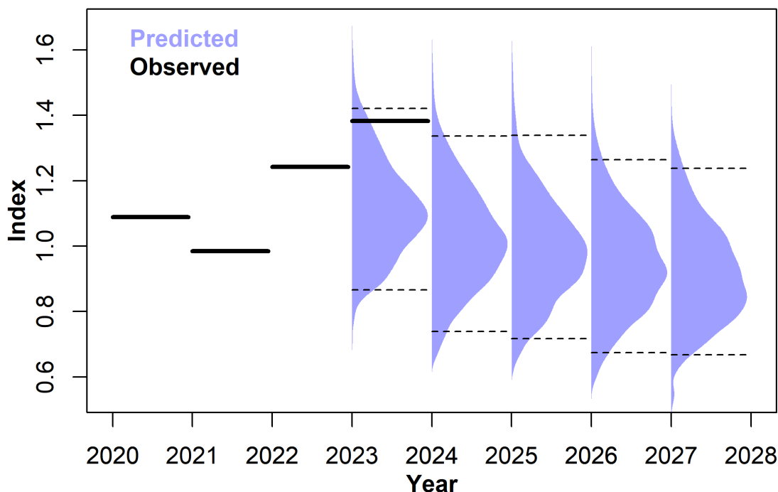
Figure 19.15.1 - Diagramme montrant l'indice combiné observé (barres horizontales noires ; 2020-2023) et les distributions de densité de l'indice combiné prédit (barres bleues ; 2023-2027) à partir des neuf OM de référence (80 simulations chacun). Les lignes noires en pointillé représentent les percentiles 2,5 et 97,5 de l'indice combiné prédit pour les neuf OM.
