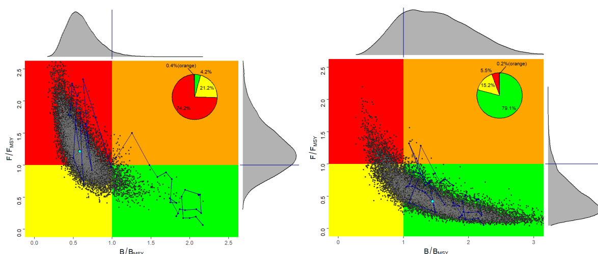
Figure 1. Trajectoires de l'état du stock de germon de la Méditerranée de B/B_{PME} et F/F_{PME} au cours du temps (1980-2022), avec l'incertitude entourant l'estimation actuelle (diagrammes de Kobe) pour le modèle bayésien de production excédentaire. Le diagramme circulaire inséré indique la probabilité que le stock se situe dans chaque quadrant de couleur de Kobe, pour les scénarios 1 (gauche) et 2 (droite). Les distributions de probabilité indiquées sur chaque axe représentent l'incertitude entourant B/B_{PME} et F/F_{PME} actuelles.
