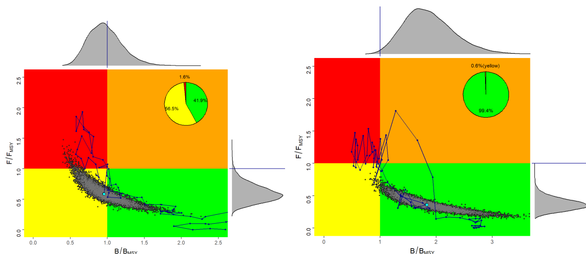
Figure 1. Diagramme de phase de Kobe pour le stock de voilier de l'Atlantique Ouest (panneau de gauche) et de l'Est (panneau de droite). Les points noirs et les lignes continues indiquent la trajectoire de l'état du stock, le point bleu indiquant la dernière année (2021), les points gris étant les interactions pour la dernière année avec les distributions marginales tracées sur l'axe latéral.
