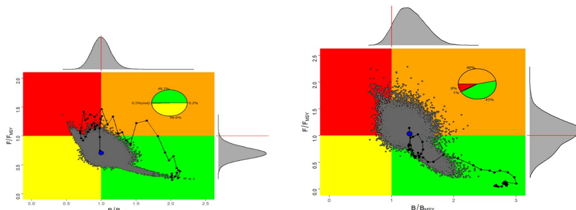
Figure 1. Diagramme de Kobe pour l'état du stock de requin peau bleue de l'Atlantique Nord (à gauche) et Sud (à droite) en 2021, estimé lors de l'évaluation des stocks (Anon. 2023d). Les lignes indiquent la trajectoire de l'état du stock à partir de 1971. Les diagrammes circulaires insérés indiquent la probabilité que le stock se situe dans chaque quadrant de couleur de Kobe.
