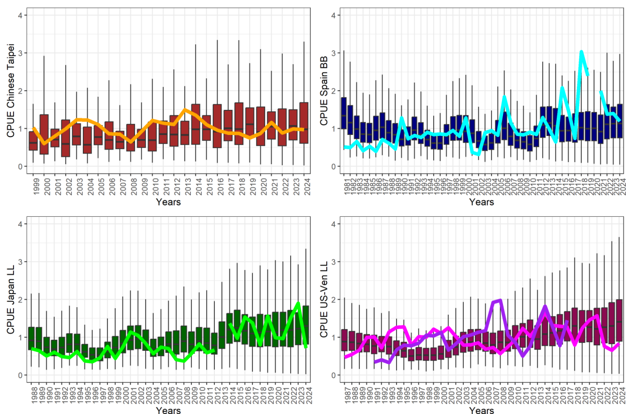
Figure 19.5.2 Trajectoires des CPUE simulées dans la MSE (diagrammes en boîte à moustaches) et CPUE standardisées actualisées (lignes). Le Taipei chinois-LL (orange), l'UE-Espagne-BB (bleu), le Japon-LL (vert) et les États-Unis-LL (rose) ont tous été mis à jour jusqu'en 2024 et le Venezuela-LL (violet) n'a pas été mis à jour depuis 2017.
