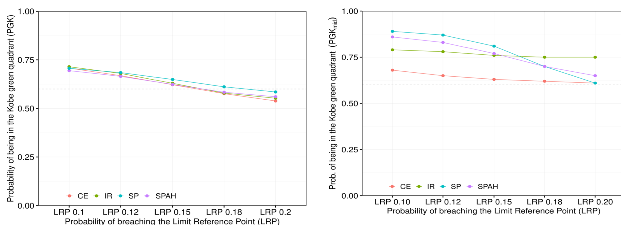
Figure 1. Relation de compromis entre la probabilité de dépasser le point de référence limite (LRP) et la probabilité de se situer dans le quadrant vert de Kobe (PGK) au cours de la période de projection de 30 ans (panneau de gauche) et à moyen terme (panneau de droite) pour les quatre CMP. Chaque ligne indique la performance de PGK au fur et à mesure que le risque de dépasser le LRP augmente de 10% à 20. La ligne horizontale en pointillés signale la PGK=60%, le niveau minimum fixé dans la Rec. 24-04 .
