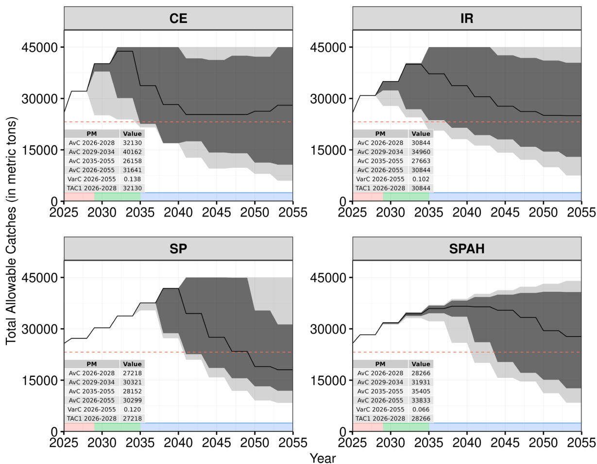
Figure 19.42.4. Projection du TAC pour le listao de l'Atlantique Ouest dans le cadre de quatre CMP, projetées pour la période 2026-2055. La ligne noire représente la trajectoire médiane, tandis que les zones ombrées correspondent aux quantiles de 80% et 95% respectivement. La ligne horizontale en pointillés rouges indique la moyenne des captures des cinq dernières années de la période historique. Les barres colorées en bas indiquent la référence de la période de projection temporelle (couleur rouge : courte ; couleur verte : moyenne ; couleur bleue : longue).
