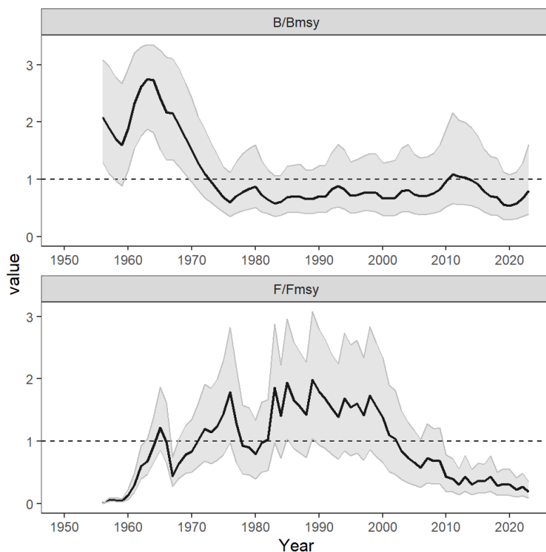
Figure 2. Trajectoires de la biomasse par rapport à B_{PME} ( B/B_{PME} ) à la fin des années et de la mortalité par pêche par rapport à F_{PME} ( F/F_{PME} ) pour le cas de base du modèle final pour le makaire blanc de l'Atlantique ; la zone ombrée indique les limites de CRI à 95%.
