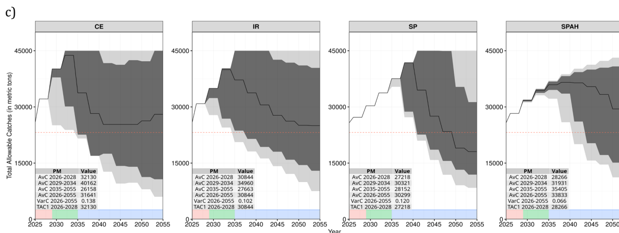
Figure 3. Trajectoire de : a) la mortalité par pêche ( F ) par rapport à F_{PME} (rangée supérieure), b) de la biomasse du stock reproducteur ( SSB ) par rapport à SSB_{PME} (rangée du milieu) et c) du TAC (en tonnes, rangée inférieure) pour les quatre CMP finales. Les résultats sont résumés pour tous les modèles opérationnels de référence. La ligne noire représente la trajectoire de la médiane, tandis que les zones ombrées correspondent aux quantiles de 80% et 95% respectivement. La ligne rouge horizontale en pointillés indique dans a) la F_{PME} , b) la SSB_{PME} et c) les captures moyennes pour les 5 dernières années de la période historique (2020-2024). Les barres rouges représentent la période courte, les barres vertes la période moyenne et les barres bleues la période longue. Les tableaux en encart dans c) indiquent les véritables TAC de 2026-28 pour chaque CMP (TAC1).
