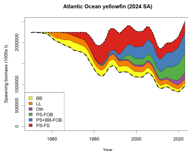
Figure 2. Les diagrammes d'impact représentent l'impact relatif de chaque engin sur la biomasse du stock reproducteur. Les zones colorées représentent les augmentations de la biomasse reproductrice prévues par le modèle lorsque les captures de chaque engin sont éliminées des captures historiques. La biomasse reproductrice non pêchée estimée (ligne pointillée) varie en fonction des écarts de recrutement. La trajectoire historique de la SSB, estimée par le modèle d'évaluation des stocks, est indiquée par une ligne en pointillés. Le code PS FOB représente les pêcheries de senneurs opérant sous des FOB/dispositifs de concentration du poisson (DCP). Le code PS+BB-FOB indique que ces flottilles de senneurs ont opéré en association avec des canneurs (BB) dans le passé. « Banc libre » fait référence aux opérations de pêche à la senne sur bancs libres.
