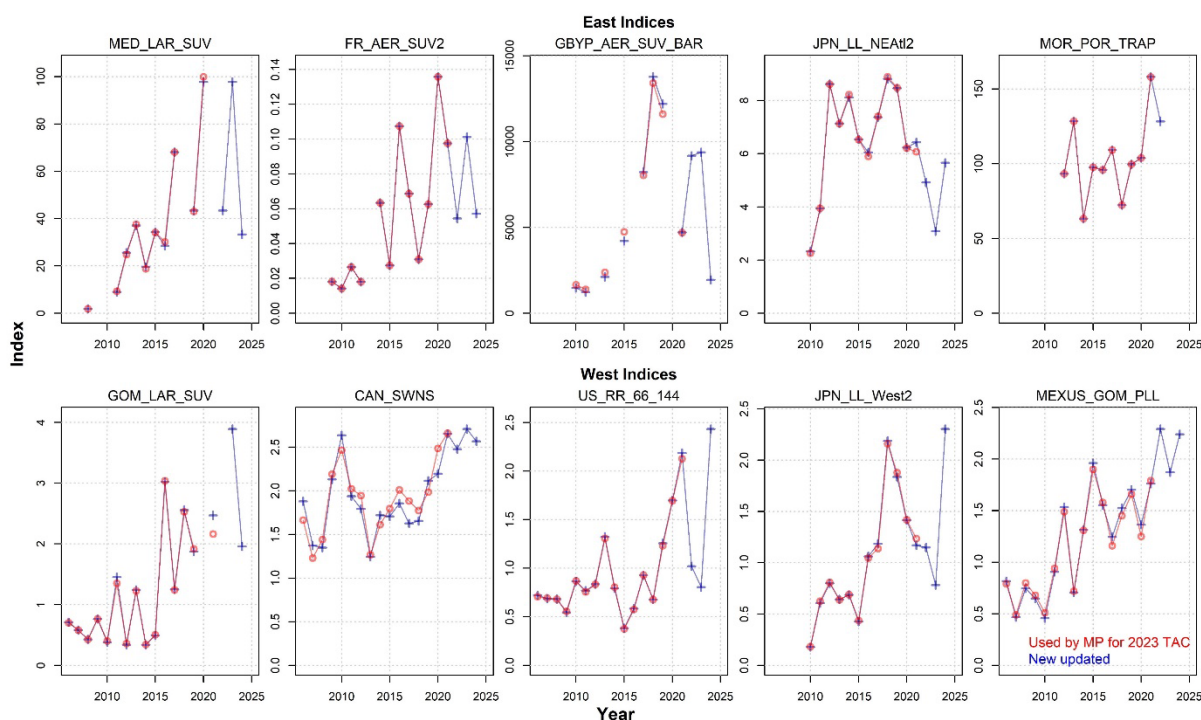
Figure 19.11.4. Diagramme des indices utilisés dans le calcul de la MP de 2022 (en rouge) et des nouveaux indices actualisés (en bleu) qui ont été rééchelonnés par le facteur k et utilisés dans les calculs de la MP pour les TAC de 2026-2028. Les valeurs en rouge sont les indices originaux utilisés pour déterminer le TAC de 2023-2025 et dans le conditionnement de la MSE et les valeurs en bleu sont de strictes actualisations des indices jusqu'en 2024 compris à utiliser dans les calculs du TAC 2026-2028. Au cours des trois dernières années, les points de données des madragues du Maroc-Portugal pour 2023 et 2024 n'ont pas été utilisés et le point de données de l'indice de la prospection larvaire dans le golfe du Mexique pour 2022 n'était pas disponible.
