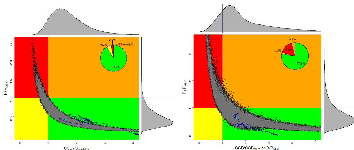
Figure 1. Diagramme de Kobe pour l'état du stock de listao de l'Atlantique Ouest (à gauche) et Est (à droite) en 2020, estimé lors de l'évaluation des stocks de 2022. Le diagramme supérieur représente la distribution de fréquence lissée des estimations de SSB_{2020}/SSB_{PME} ou B_{2020}/B_{PME} pour 2020, alors que le diagramme de droite représente la distribution de fréquence lissée des estimations de F_{2020}/F_{PME} pour 2020. Les diagrammes circulaires insérés indiquent la probabilité que le stock se situe dans chaque quadrant de couleur de Kobe. La ligne indique la trajectoire de l'état du stock à partir de 1952 pour les stocks de l'Ouest et de l'Est.
