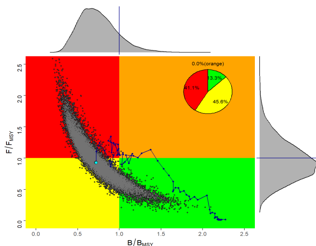
Figure 1. Diagramme de Kobe pour les trajectoires de l'état du stock d'espadon de la Méditerranée pour les distributions a posteriori combinées en 2018, estimées lors de l'évaluation du stock en 2020. Le diagramme circulaire inséré indique la probabilité que le stock se situe dans chaque quadrant de couleur de Kobe. Les distributions de probabilité indiquées sur chaque axe représentent l'incertitude entourant B/B_{PME} et F/F_{PME} actuelles. La ligne noire indique la trajectoire de l'état du stock à partir de 1950.
