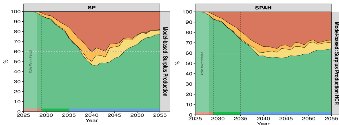
Figure 2. Diagramme temporel de Kobe montrant le pourcentage (axe vertical) des simulations de tous les modèles opérationnels de référence qui se situent dans chacun des quadrants de Kobe pour chaque année de projection (axe horizontal). Le vert indique que le stock n'est ni surexploité ni ne fait l'objet de surpêche. L'orange signifie que le stock fait l'objet de surpêche mais n'est pas surexploité. Le jaune indique que le stock est surexploité mais ne fait pas l'objet de surpêche. Le rouge signifie que le stock est à la fois surexploité et fait l'objet d'une surpêche continue. La ligne verticale délimite les différentes périodes temporelles, les barres rouges indiquant le court terme, les barres vertes le moyen terme et les barres bleues le long terme.
