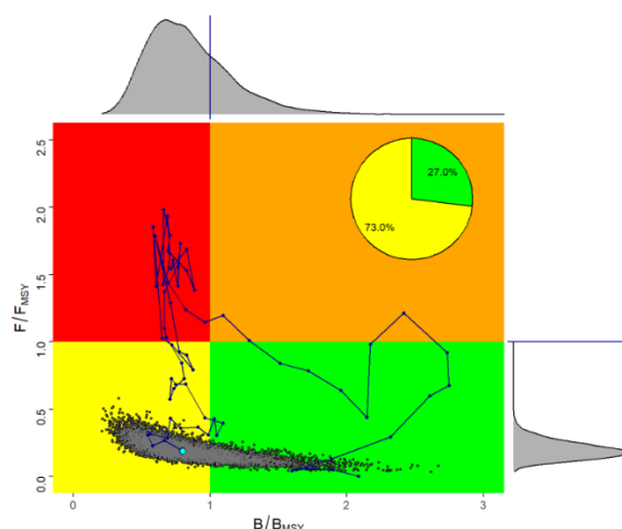
Figure 1. Diagramme de Kobe pour l'état du stock de makaire blanc/makaire épée de l'Atlantique en 2023, estimé lors de l'évaluation du stock de 2025. La ligne indique la trajectoire de l'état du stock à partir de 1956. Le diagramme circulaire inséré indique la probabilité que le stock se situe dans chaque quadrant de couleur de Kobe. Les distributions de probabilité indiquées sur chaque axe représentent l'incertitude entourant B/B_{PME} et F/F_{PME} actuelles.
