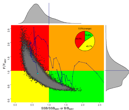
Figure 1. Diagramme de Kobe pour l'état du stock de makaire bleu de l'Atlantique en 2022, estimé lors de l'évaluation du stock de 2024 (Anon., 2024i). La ligne indique la trajectoire de l'état du stock à partir de 1952. Le diagramme circulaire inséré indique la probabilité que le stock se situe dans chaque quadrant de couleur de Kobe. Les distributions de probabilité indiquées sur chaque axe représentent l'incertitude concernant les niveaux actuels de B/B_{PME} ( SS3 , SSB/SSB_{PME} ) et de F/F_{PME} .
