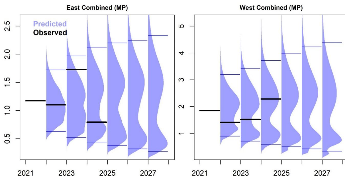
Figure 19.11.1. Diagrammes standards marginaux des indices composites observés (barres noires) et distribution des données prédites a posteriori (distribution de densité bleue) pour la grille de référence des OM (n =2304, 48 OM, 48 simulations pour chacun). Les barres bleues représentent les intervalles de 95 %. Le point de données des madragues du Maroc-Portugal pour 2024 n’a pas été utilisé en raison de changements dans la distribution temporelle des captures qui ont créé des problèmes insolubles pour la standardisation de l’indice existant.
