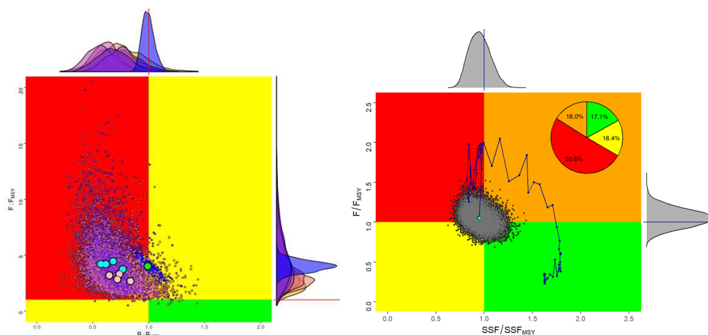
Figure 1. Diagramme de Kobe pour l'état du stock de requin-taupe bleu de l'Atlantique Nord (à gauche) et Sud (à droite) en 2015 et 2023, estimé lors des évaluations des stocks de 2017 et 2025, respectivement. Les lignes indiquent la trajectoire de l'état des stocks à partir de 1971. Les graphiques circulaires insérés dans le diagramme du Sud indiquent la probabilité que le stock se situe dans chaque quadrant de couleur de Kobe.
