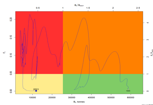
Figure 1. Diagramme de Kobe représentant l'état du stock de requin-taube commun de l'Atlantique Nord-Est en 2021, estimé lors de l'évaluation du stock de 2022. La ligne indique la trajectoire de l'état du stock à partir de 1926.
