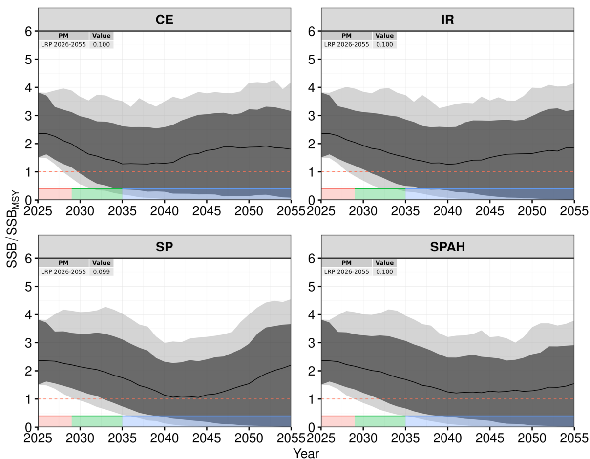
Figure 19.42.2. Projection de la biomasse du stock reproducteur par rapport à la SSB_{PME} ( SSB/SSB_{PME} ) pour le listao de l'Atlantique Ouest dans le cadre de quatre CMP, projetées pour la période 2026-2055. La ligne noire représente la trajectoire médiane, tandis que les zones ombrées correspondent aux quantiles de 80% et 95% respectivement. La ligne horizontale en pointillés rouges indique le point de référence cible ( SSB_{PME} = 1 ). Les barres colorées en bas indiquent la B_{LIM} de référence ( 0.4 * SSB_{PME} ) pour chaque période de projection temporelle (couleur rouge : courte ; couleur verte : moyenne ; couleur bleue : longue).
