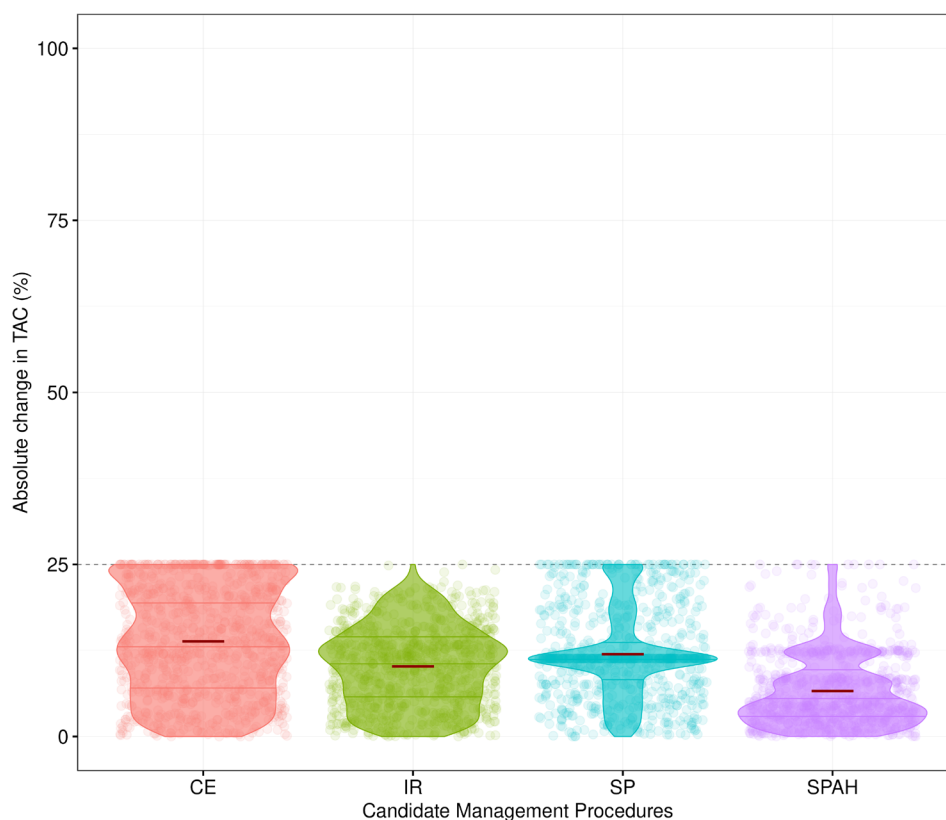
Figure 4. Diagramme en violon pour le changement du TAC entre les cycles de gestion. La largeur du diagramme en violon indique la proportion de points de données qui se trouvent dans chaque région du diagramme (c'est-à-dire que les zones larges du diagramme indiquent un nombre relativement important de points de données dans cette région, tandis que les zones étroites du diagramme indiquent peu de points de données). Les lignes à l'intérieur des diagrammes en violon indiquent les percentiles 25, 50 et 75, et la ligne rouge la moyenne des distributions.
