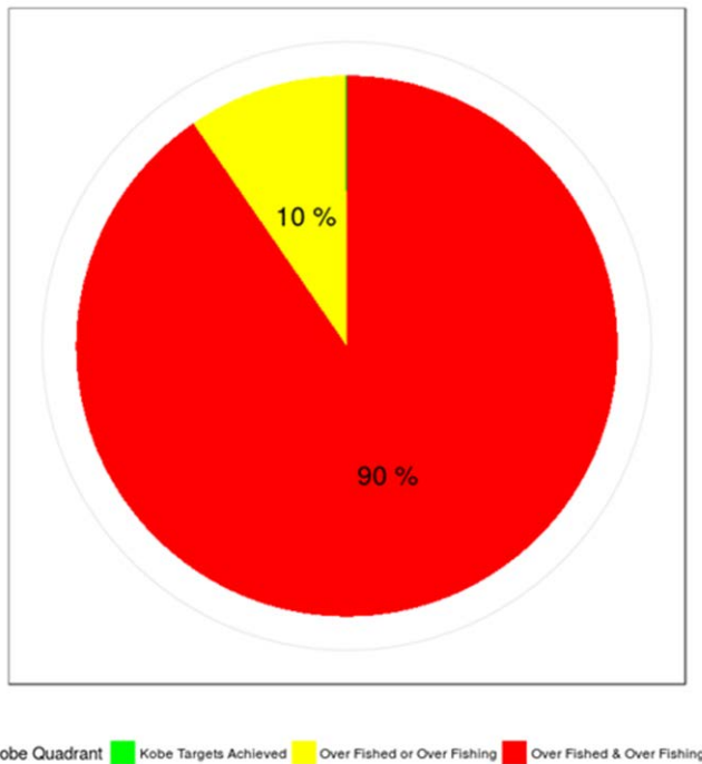
SMA-figure 5. Diagramme de Kobe résumant l'état du stock (pour 2015) pour le requin-taupo bleu de l'Atlantique Nord d'après les modèles de production de type bayésien (4 scénarios BSP2JAGS et 4 scénarios JABBA) et 1 modèle structuré par âge, basé sur les tailles (SS3). La probabilité de se situer dans le quadrant vert est inférieure à 0,5 %.
