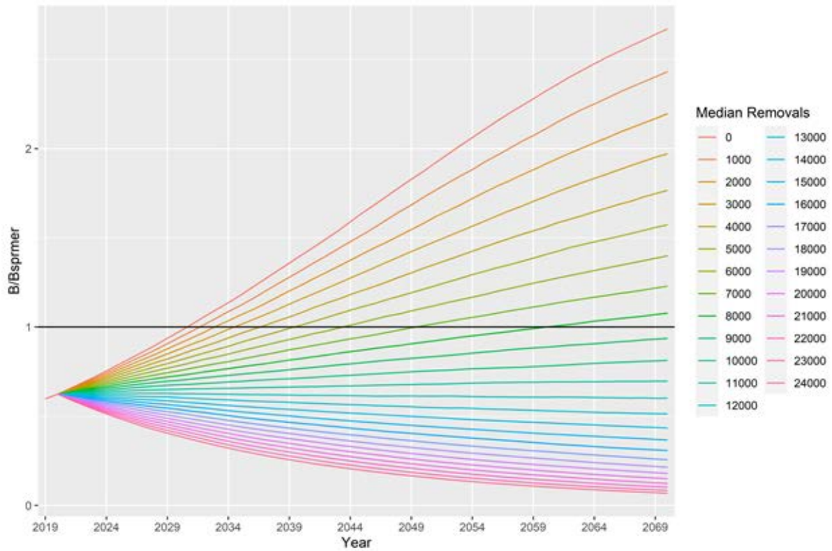
POR-figure 3. Requin-taupe commun de l'Atlantique Nord-Ouest - Abondance relative prédite pour des ponctions annuelles allant de 0 à 24.000 animaux pour le stock du Nord-Ouest, exprimée par le ratio biomasse/biomasse à SPR_{MER} (approximation de B_t/B_{PME} ) pour le cas de base de l'ICM. La ligne horizontale indique le point de référence et les projections s'étendent sur 50 ans. Les ponctions moyennes de 2016 à 2018 ont été supposées pour 2019 et 2020 et la projection commence en 2021.
