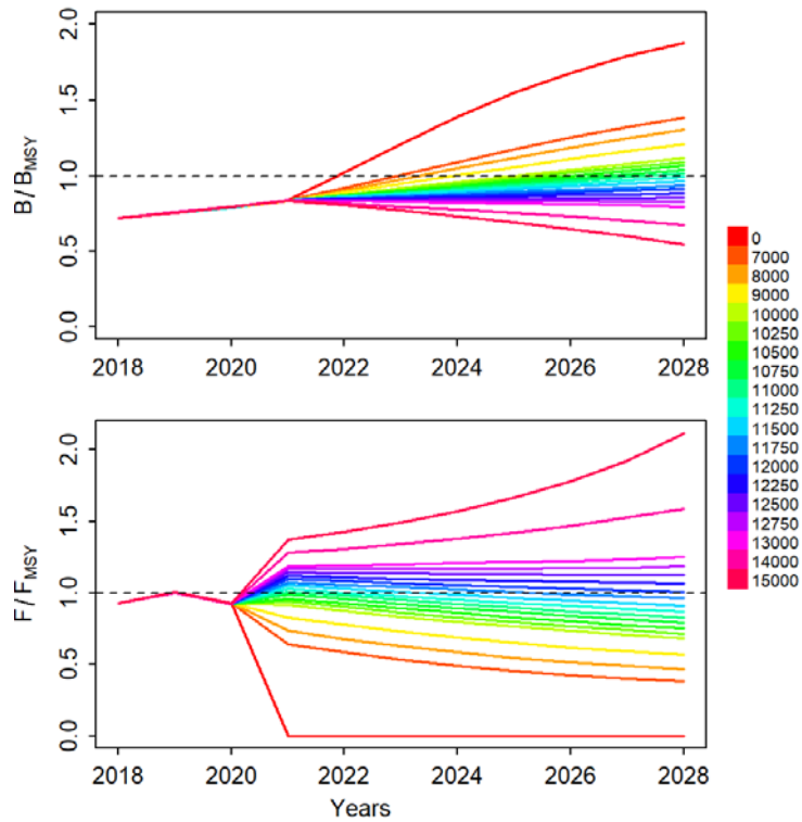
SWO-MD-figure 5. Tendances de la biomasse du stock (au début de l'année, panneau supérieur, B/B_{PME} ) et de la mortalité par pêche (à la fin de l'année, panneau inférieur, F/F_{PME} ) relatives et projetées de l'espadon de la Méditerranée, selon différents scénarios de TAC (0 - 15.000 t), sur la base des projections combinées des scénarios du modèle JABBA. Chaque ligne représente la médiane des 30.000 itérations MCMC par année projetée.
