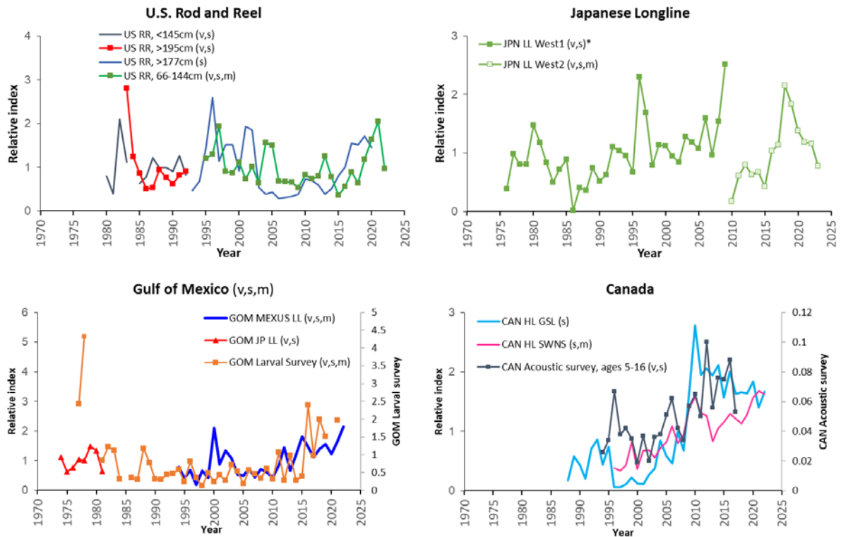
BFTW-figure 2. Indices d'abondance relative pour le thon rouge de l'Ouest. Les indices portant un « s » ont été utilisés dans Stock Synthesis, ceux portant un « v » sont ceux utilisés dans la VPA et les indices portant un « m » sont ceux utilisés dans la procédure de gestion. (*) Le faible point de données de 1986 de la palangre japonaise dans l'Atlantique Ouest a été supprimé dans les modèles de Stock Synthesis.
