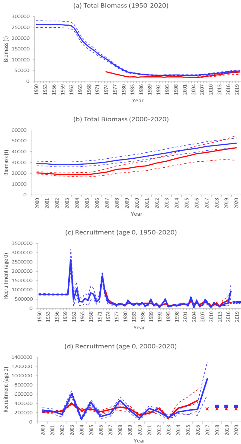
BFTW-figure 3. Estimations (a) de la biomasse totale des stocks pour 1950-2020 et (b) pour 2000-2020, (c) du recrutement (âge 0) pour 1950-2020 et (d) pour 2000-2020 pour le cas de base des modèles VPA (rouge) et Stock Synthesis (bleu) de l'évaluation de 2021. Les lignes en pointillé indiquent les intervalles de confiance de 80%. Les estimations du recrutement pour les années récentes (2017-2020 pour la VPA ; 2018-2020 pour Stock Synthesis) ont été remplacées par le recrutement moyen des six récentes années (2012-2017).
