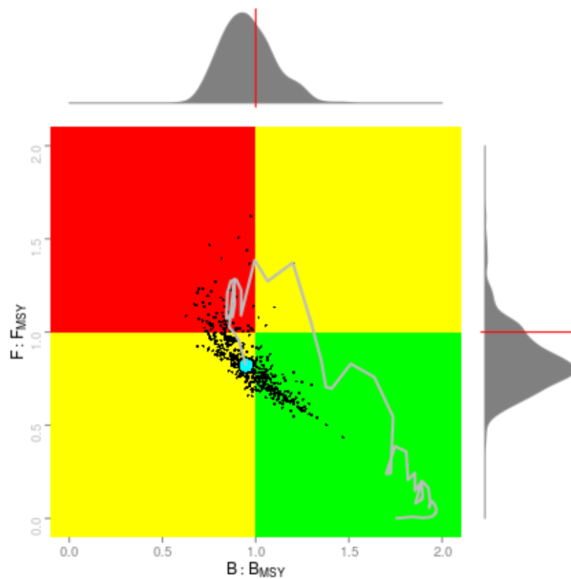
SWO-ATL-Figura 15. Diagrama de Kobe para el modelo de referencia ASPIC para el pez espada del Atlántico sur. Los rombos muestran la incertidumbre y la línea representa la trayectoria del estado del stock para F/F_{RMS} y B/B_{RMS} , 1950-2011.
