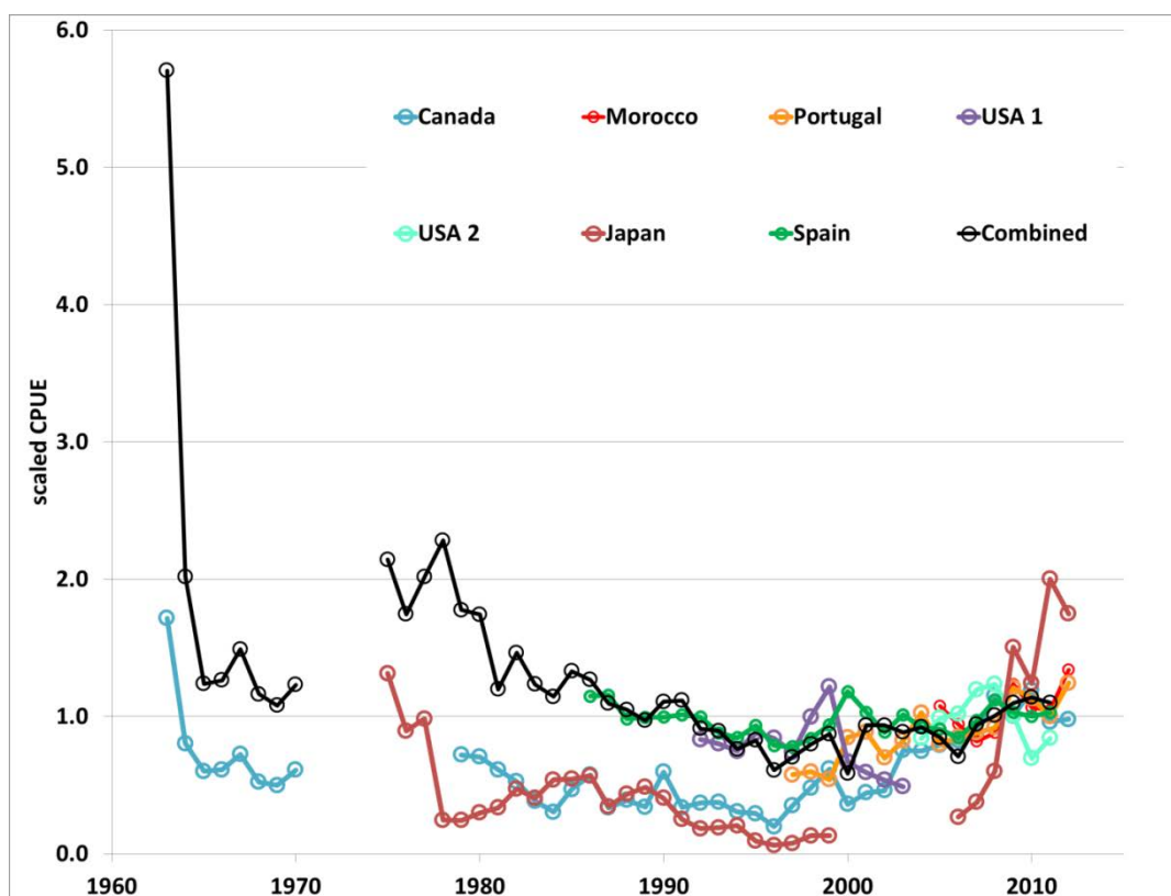
SWO-ATL-Figura 4. Series de CPUE estandarizadas facilitadas por las CPC para el pez espada del Atlántico norte e índice combinado del caso base del modelo de producción. Las series de CPUE fueron escaladas a su media para los años de solapamiento.
