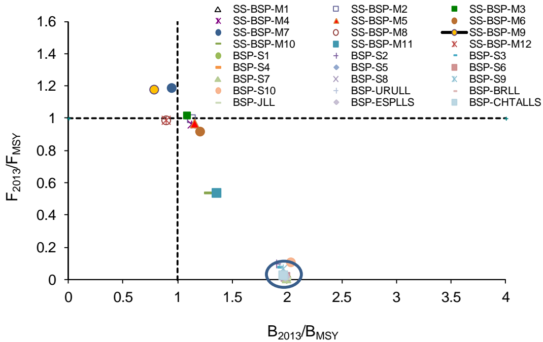
SHK-Figura 8. Diagramas de fase que resumen los resultados del escenario para la actual (para 2013) situación del stock de tinterera del Atlántico sur (BSH). BSP = modelo de producción excedente bayesiano; SS -BSP = modelo de producción excedente bayesiano de estado-espacio. El círculo indica la situación común para varios ensayos de BSP.
