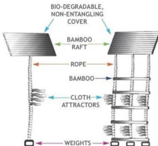
Figura. Ejemplo de un DCP biodegradable y no enmallante
