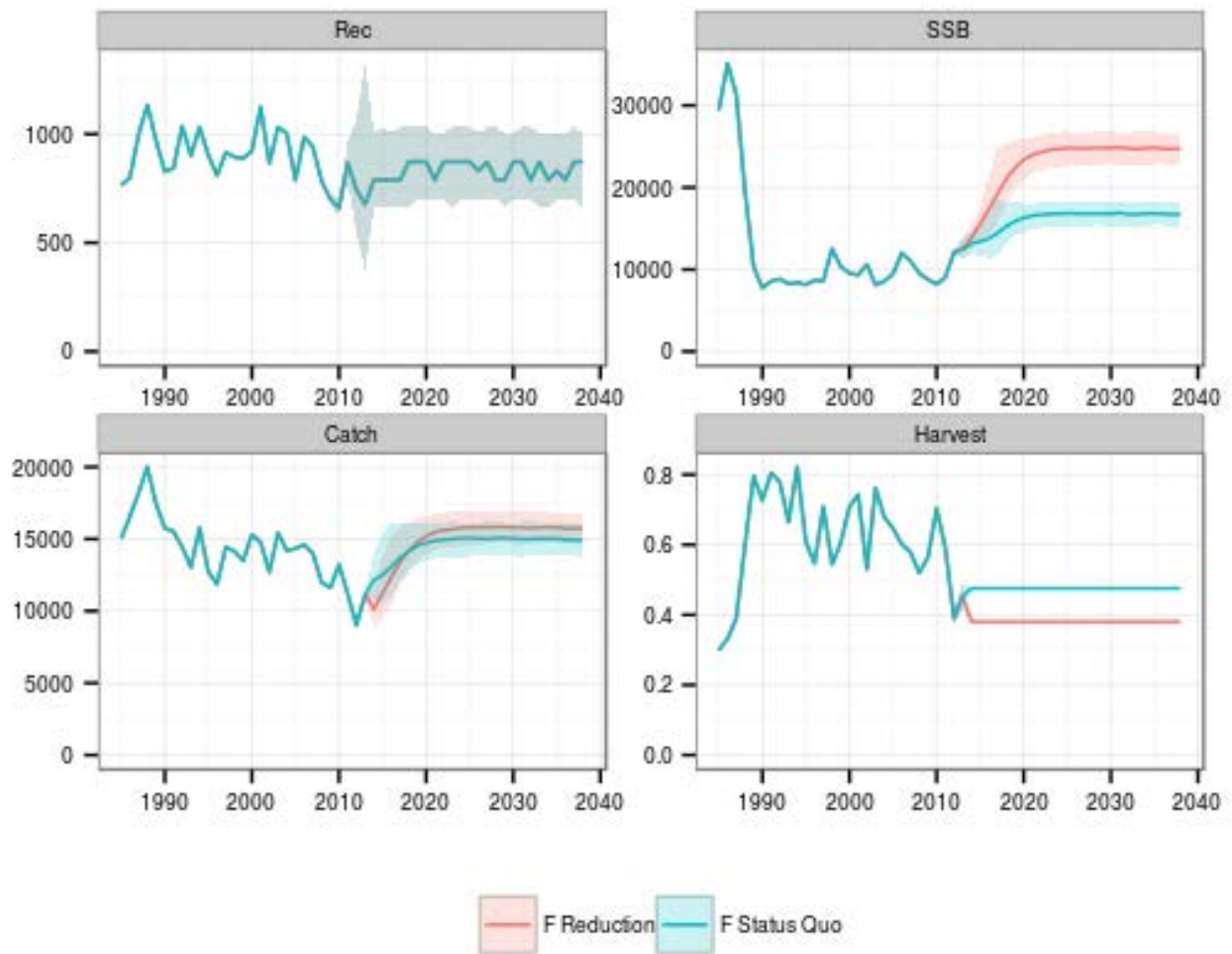
SWO-MED-Figura 10. Proyecciones basadas en un patrón de selección mixto (50:50 actual y mesopelágico) y dos niveles de F (captura) diferentes; statu quo (azul) y 80% del actual (rojo). Las estimaciones se basan en la evaluación XSA.
