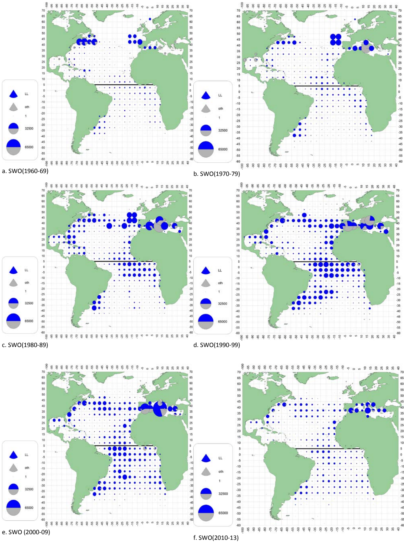
SWO-ATL-Figura 1. Distribución geográfica de la captura acumulada (t) de pez espada, por arte, en la zona del Convenio, por décadas. Los gráficos están escalados a la captura máxima observada en 1960-2013.
