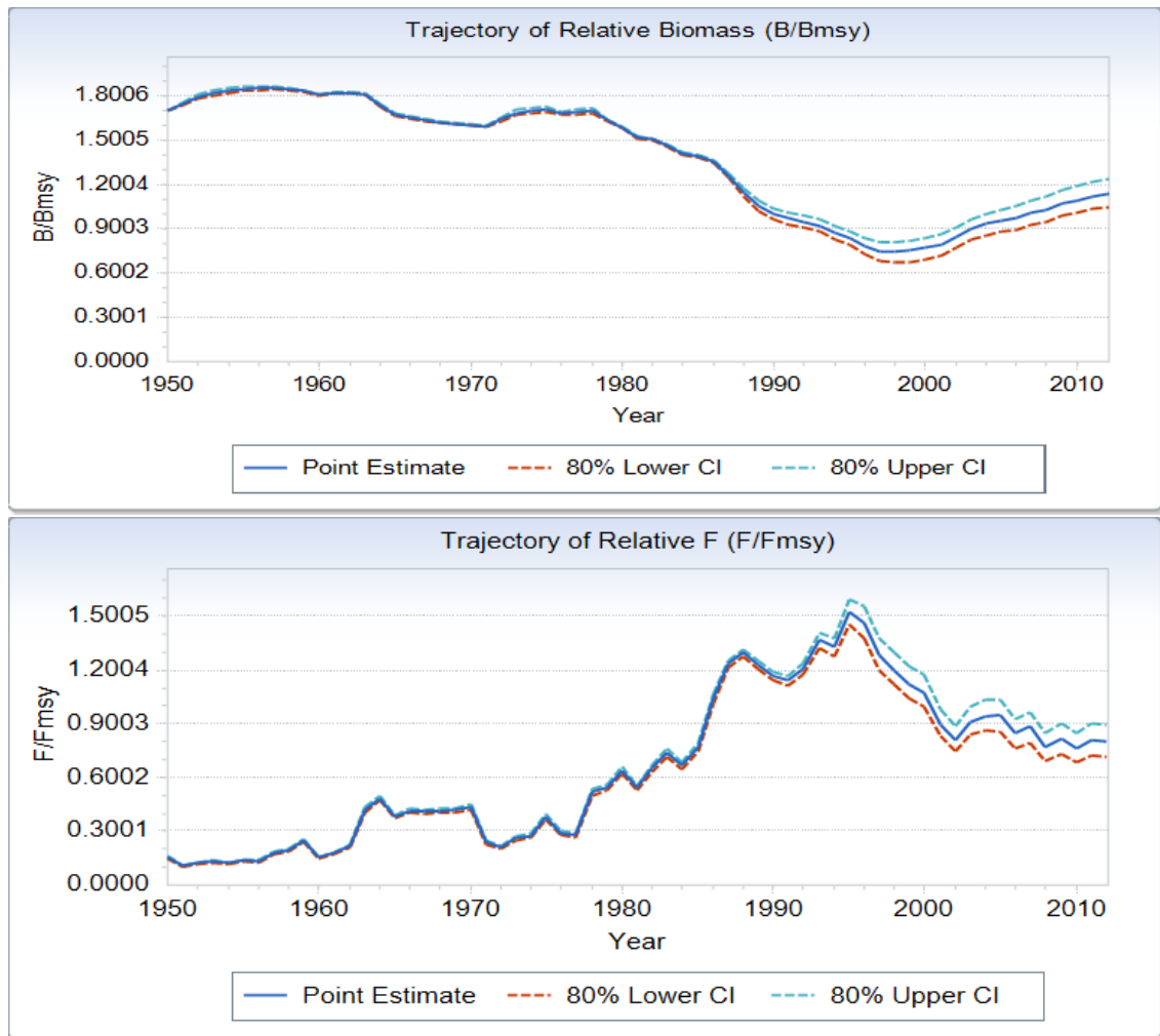
SWO-ATL-Figura 8. Resultados del caso base de ASPIC para el Atlántico norte: tendencias en las estimaciones puntuales de la biomasa (arriba) y en la mortalidad por pesca (abajo) relativas de pez espada.
