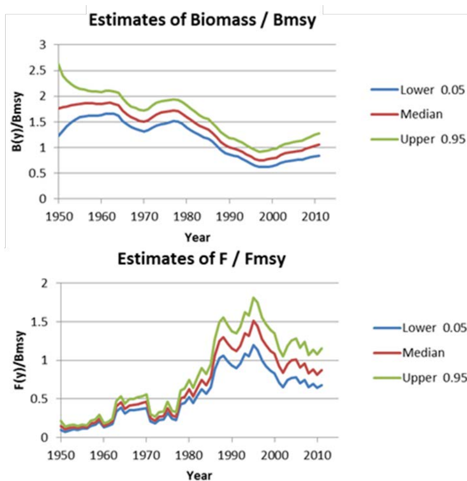
SWO-ATL-Figura 11. Diagramas de las ratios de: i) biomasa del stock respecto a B_{RMS} y ii) tasa de mortalidad por pesca respecto a F_{RMS} a partir del caso base de BSP2 para el pez espada del Atlántico norte.
