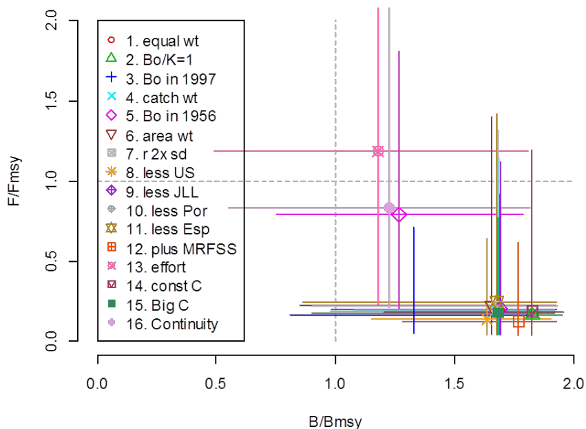
SHK-Figura 9. Para el marrajo dentado del Atlántico norte, mediana de la biomasa respecto a B_{RMS} y mediana de la mortalidad por pesca respecto a F_{RMS} , con intervalos de confianza del 80%, procedente del modelo BSP.
