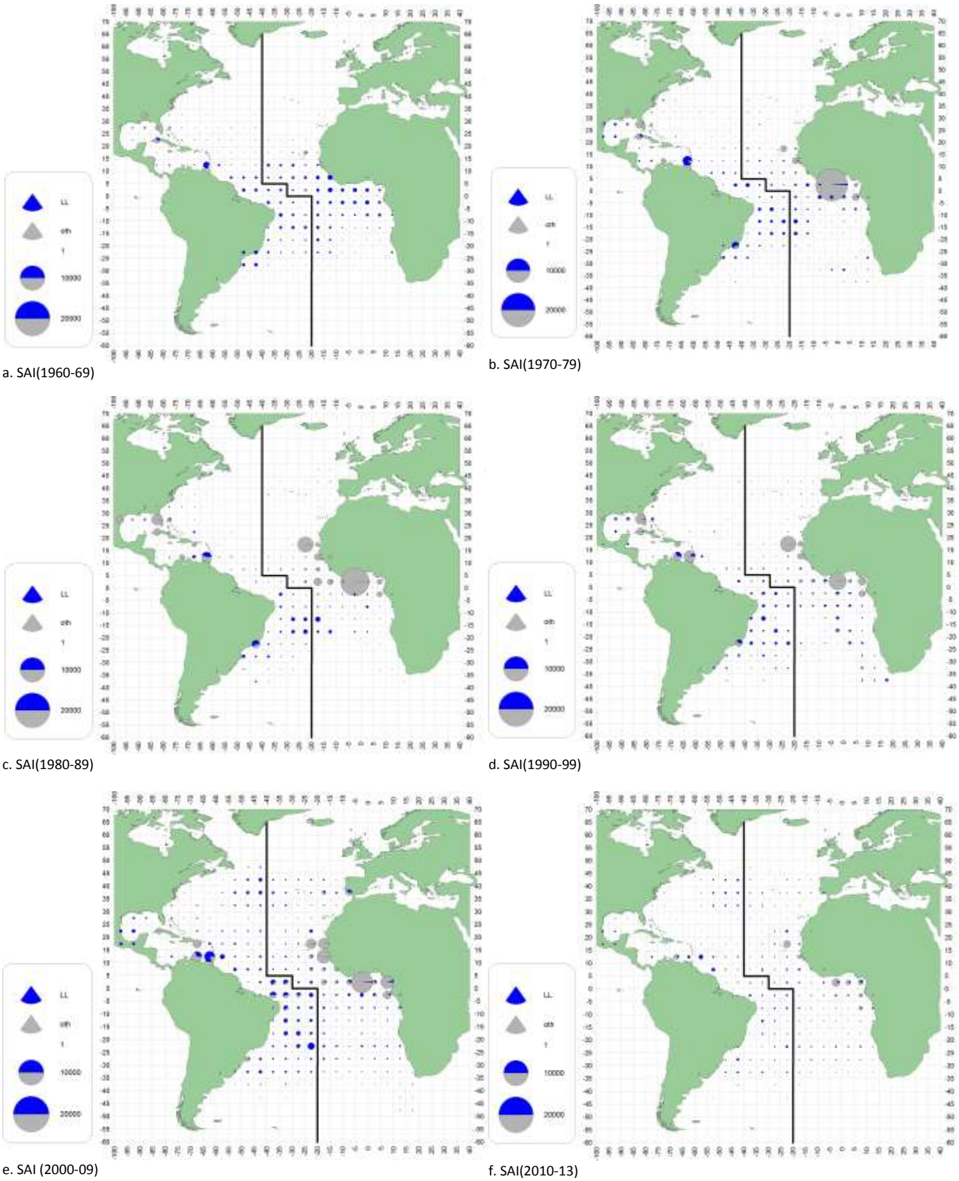
SAI-Figura 1. Distribución geográfica de las capturas medias de pez vela por artes principales y por décadas. La línea oscura indica la separación entre stocks.
