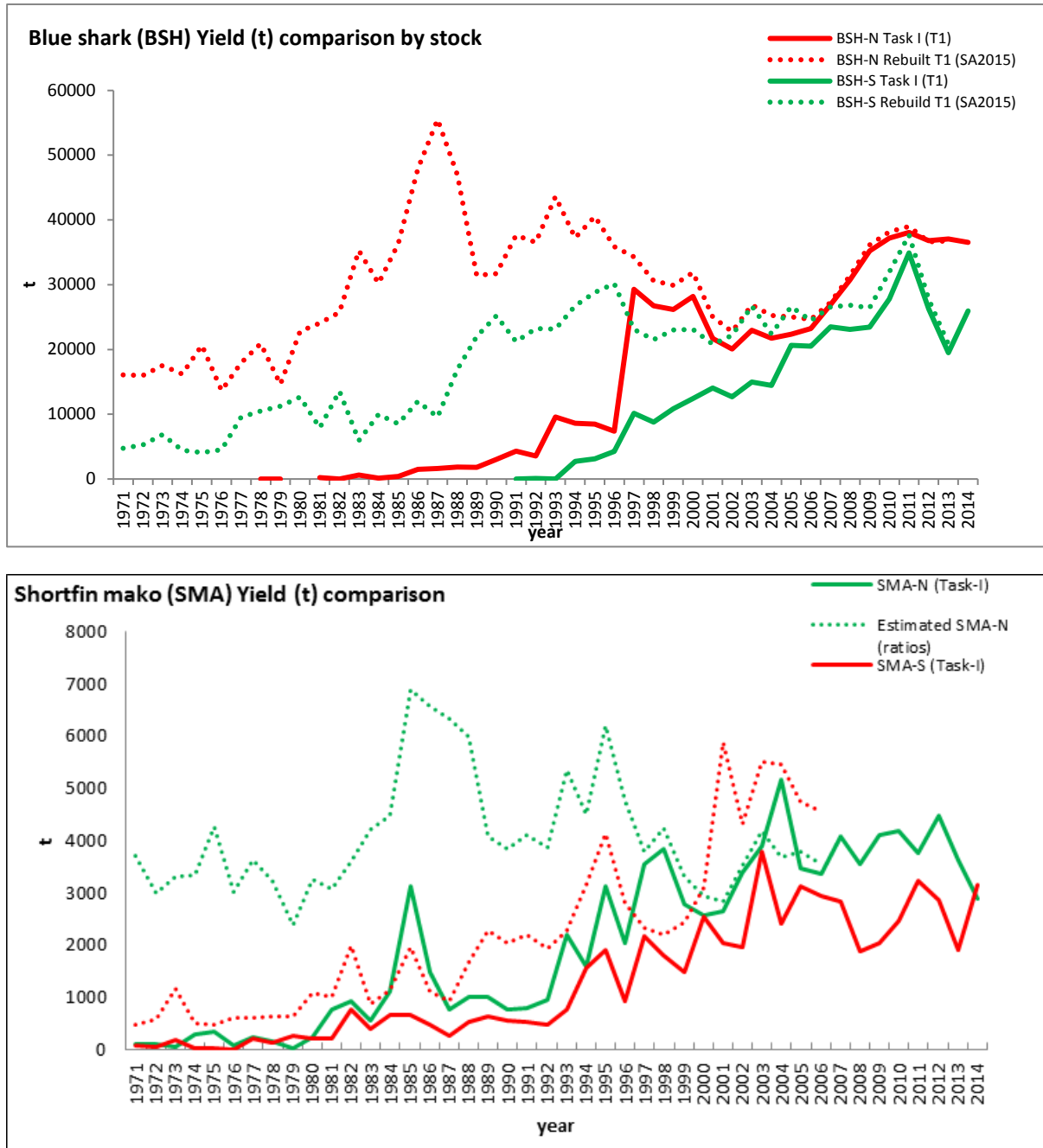
SHK-Figura 1. Capturas de tintorera (BSH) y marrajo dientoso (SMA) declaradas a ICCAT (Tarea I) y estimadas por el Comité (los desembarques de 2014 son provisionales).
