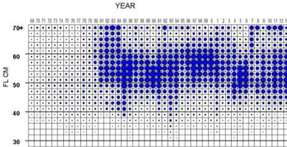
SKJ-Figura 13. Captura anual (en peso) por clase de talla del listado en el Atlántico oeste.
