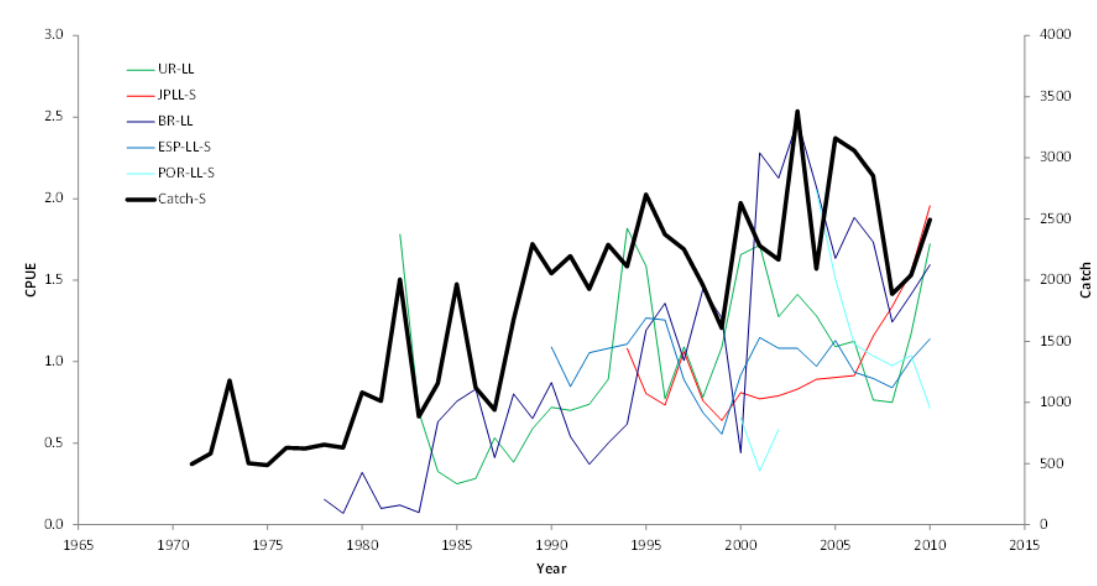
SHK-Figura 5. Capturas de marrajo sardinero del Atlántico sur e índices de abundancia introducidos en el modelo BSP.
